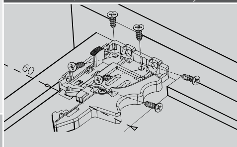
把手安装Bracket Assembly
