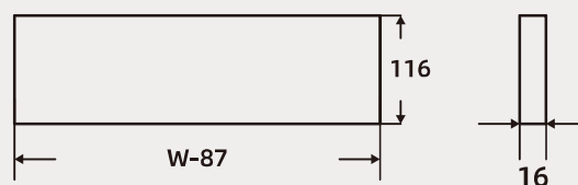
抽屉所需空间 Drawer space requirement
