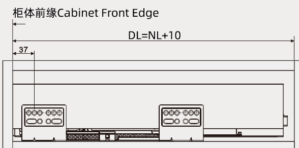
抽屉所需空间 Drawer space requirement
